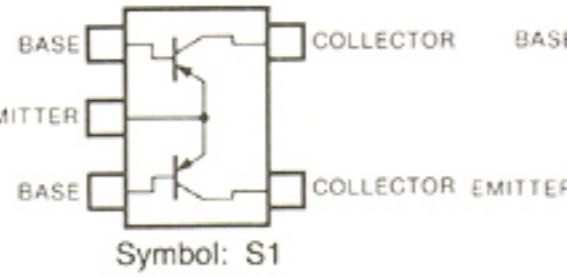
FMS1 Q20
